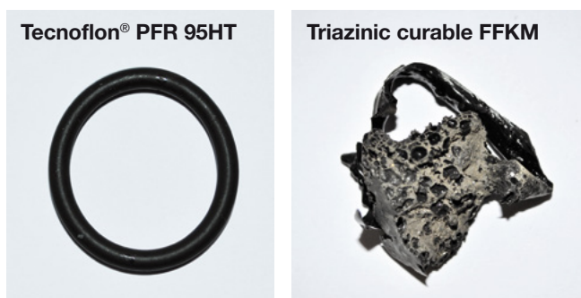
蒸汽影响: 一周放置于300°C下
