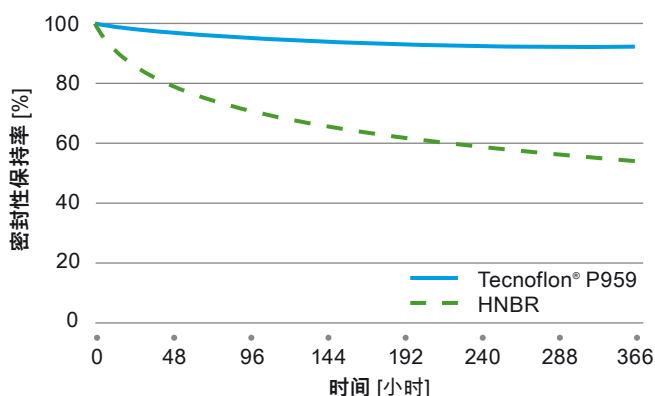
150°C下压缩应力松弛
