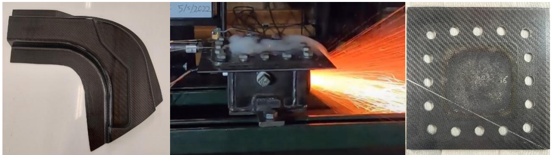
SolvaLite® 716 FR コンポーネントに対して実施された UL 2596 燃焼試験 - 前後. (写真: Solvay, PR093)
