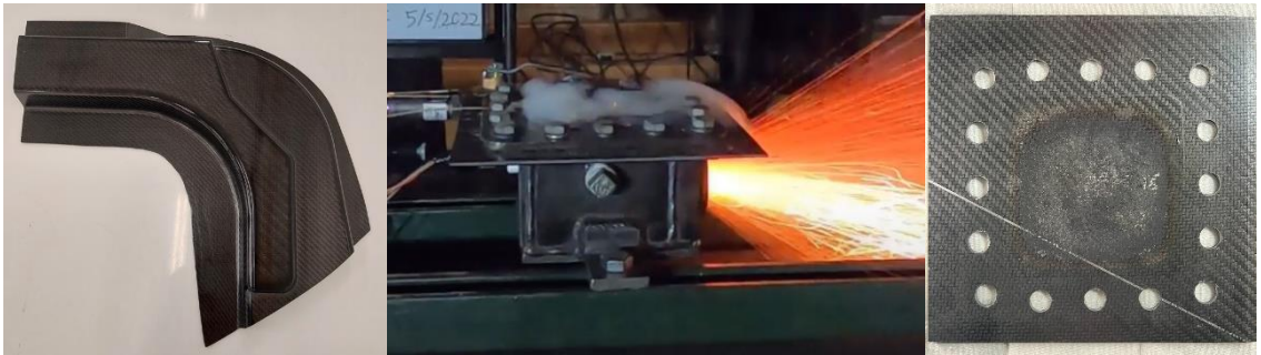
SolvaLite® 716 FR 부품에 대해 수행된 UL 2596 화염 테스트 - 전후. (사진: Solvay, PR093)
